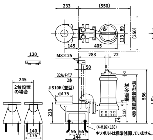
S3A65
