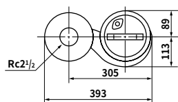
S3A65
