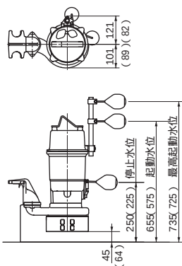
AH502W
