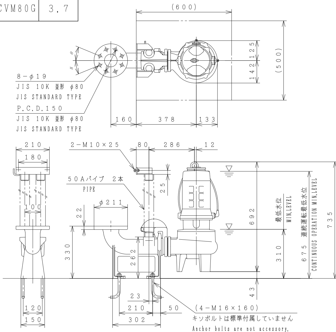
自動接続型 外形寸法図 (AUTOMATIC CONNECTION TYPE PUMP DIMENSION) 接続型番 (CONNECTION TYPE) P80B
