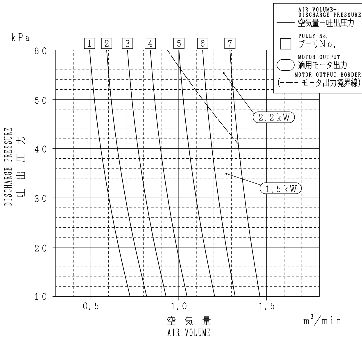
A R H 4 0 E X 性能曲線図 (PERFORMANCE CURVE)
