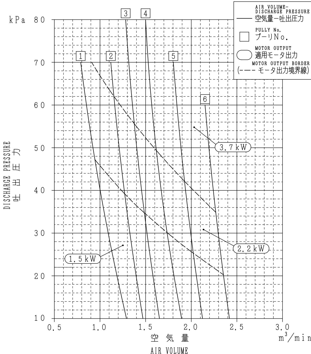
A R H 5 0 E X 性能曲線図 (PERFORMANCE CURVE)
