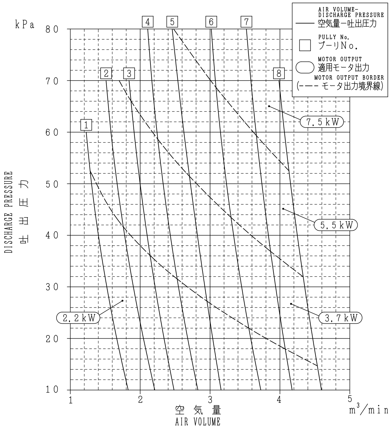
AR H 6 5 E X 性能曲線図 (PERFORMANCE CURVE)
