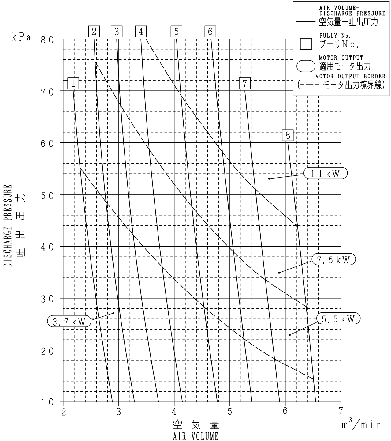
ARH80EX 性能曲線図 (PERFORMANCE CURVE)
